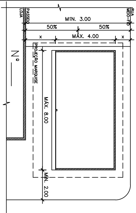
02 PLANTA BAIXA ESCALA 1:75
