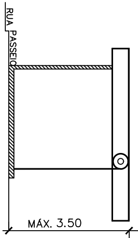
01 CORTE ESCALA 1:75
